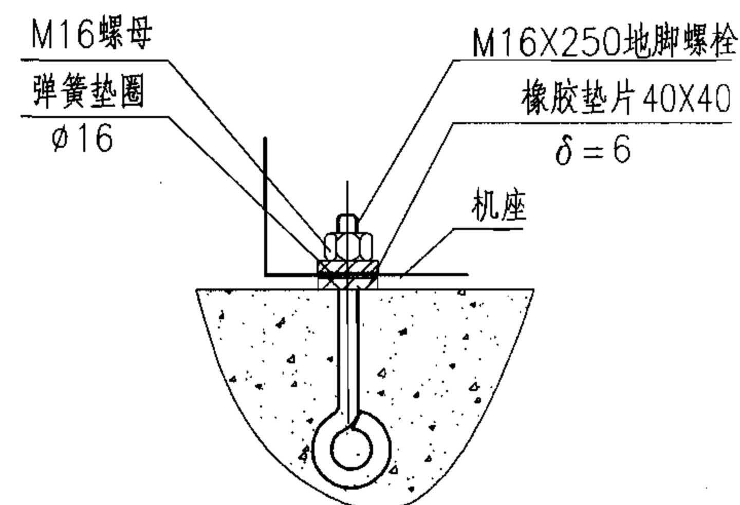
橡胶垫片安装
