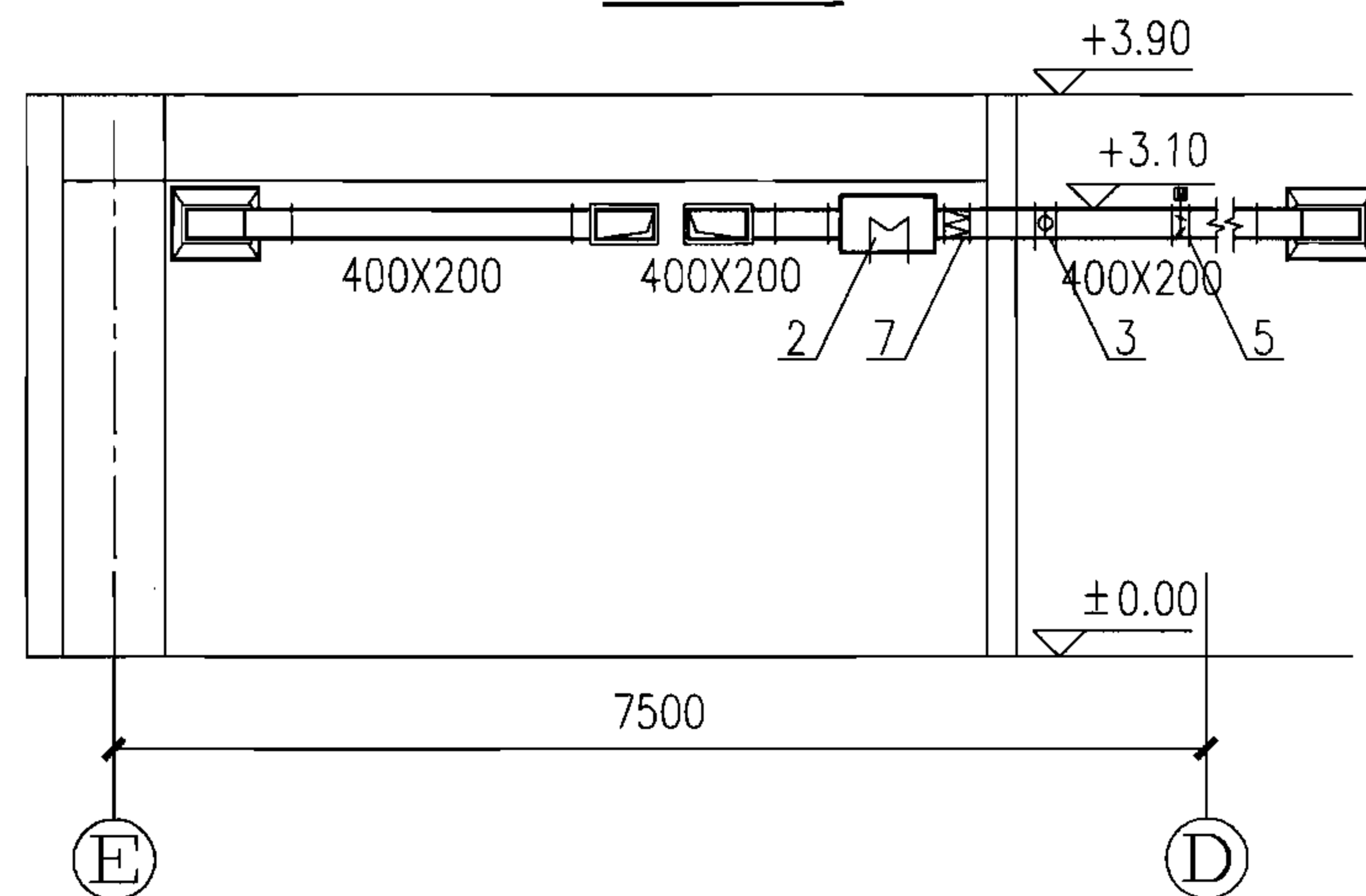
B-B剖面图
