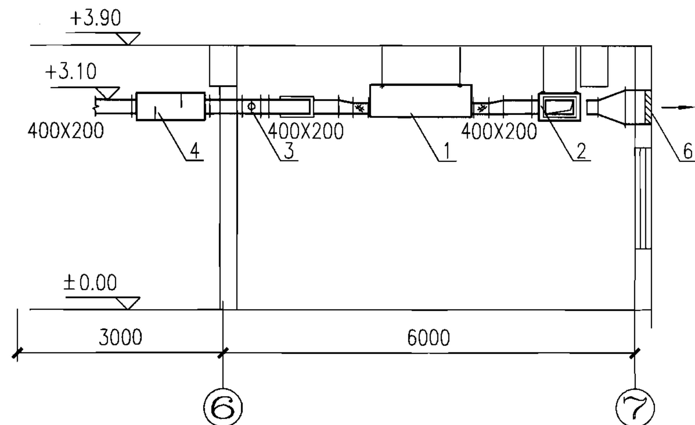
A-A剖面图
