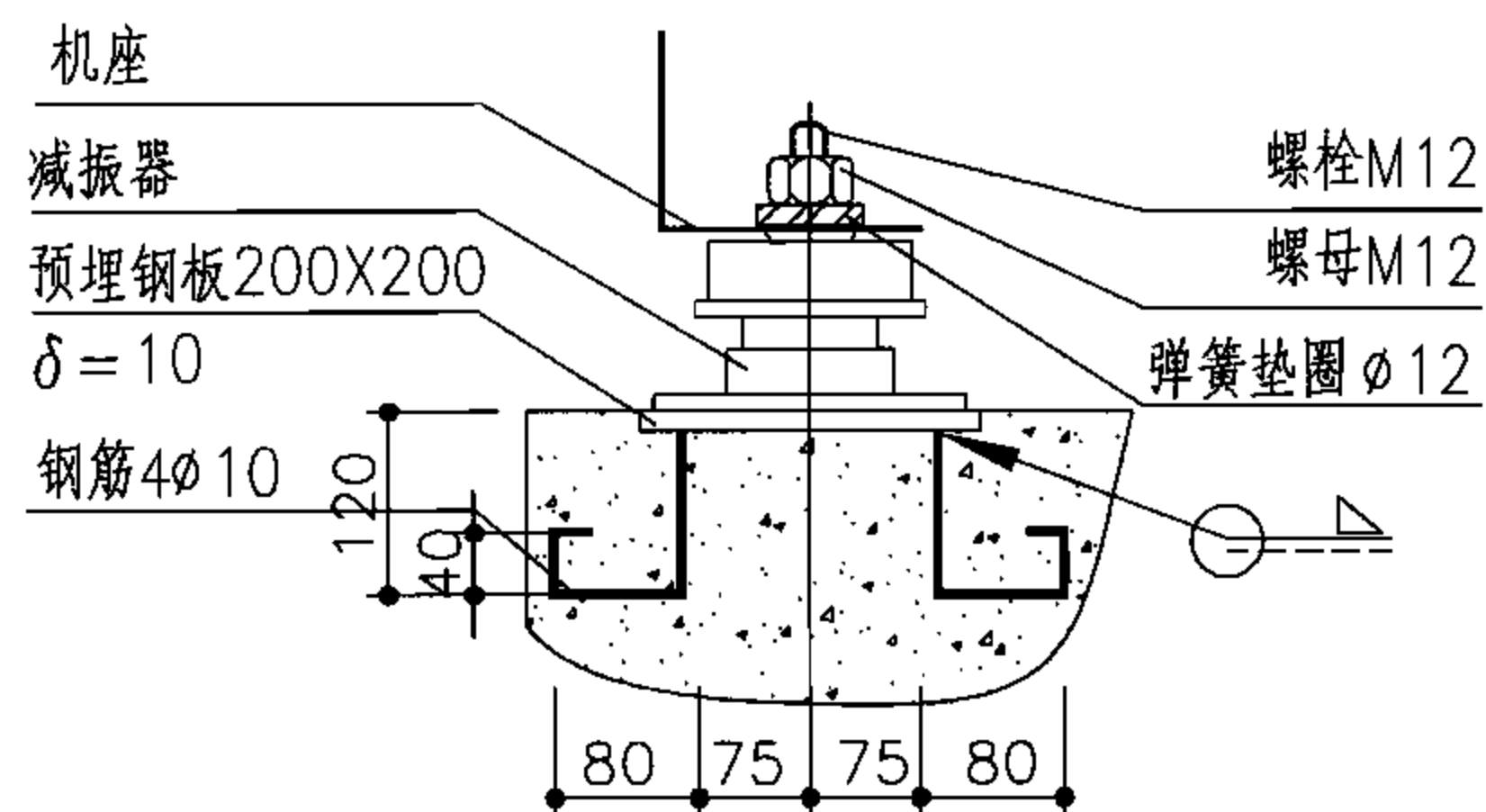
弹簧减振器安装
