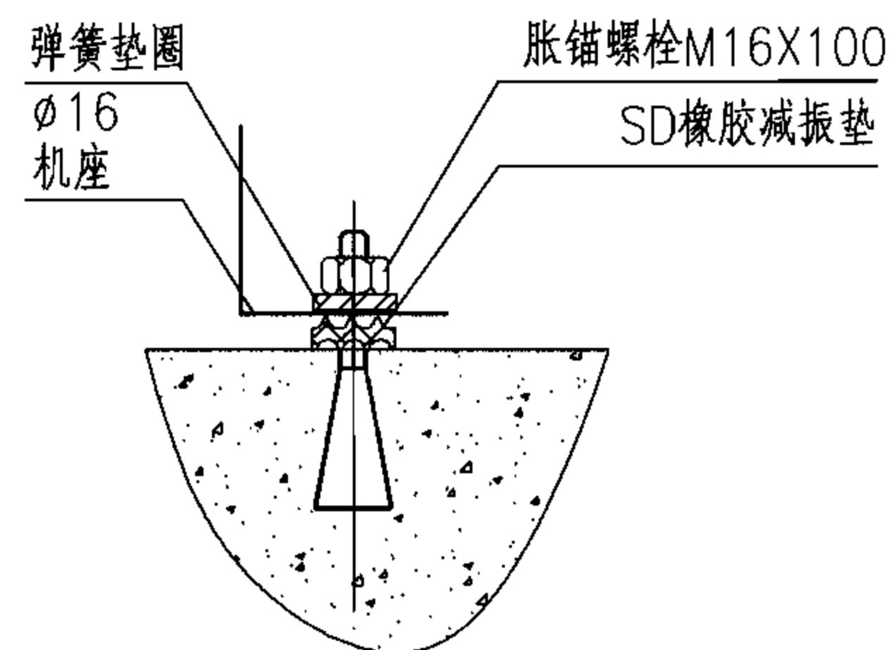
SD橡胶减振垫安装
