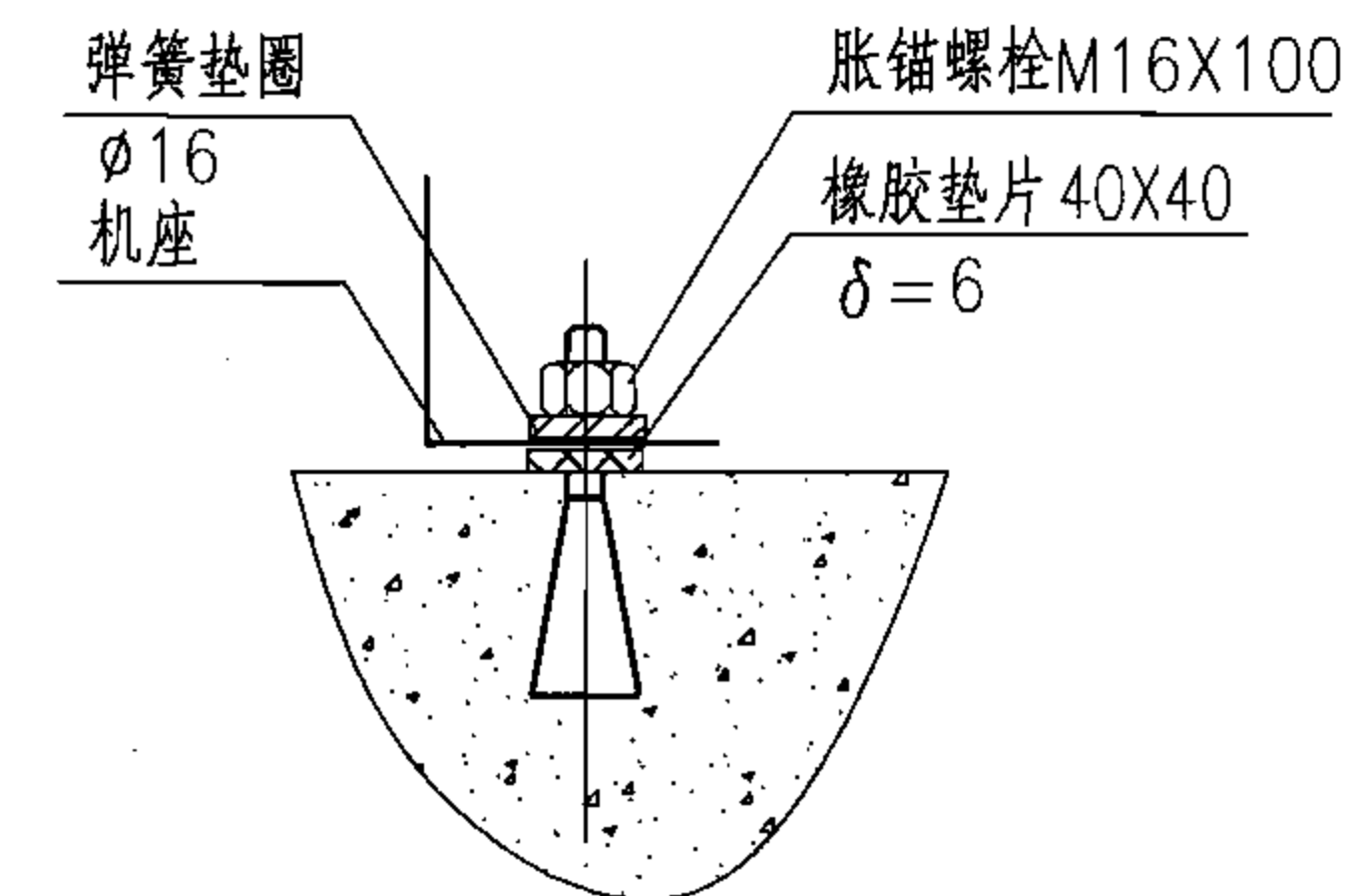
橡胶垫片安装
