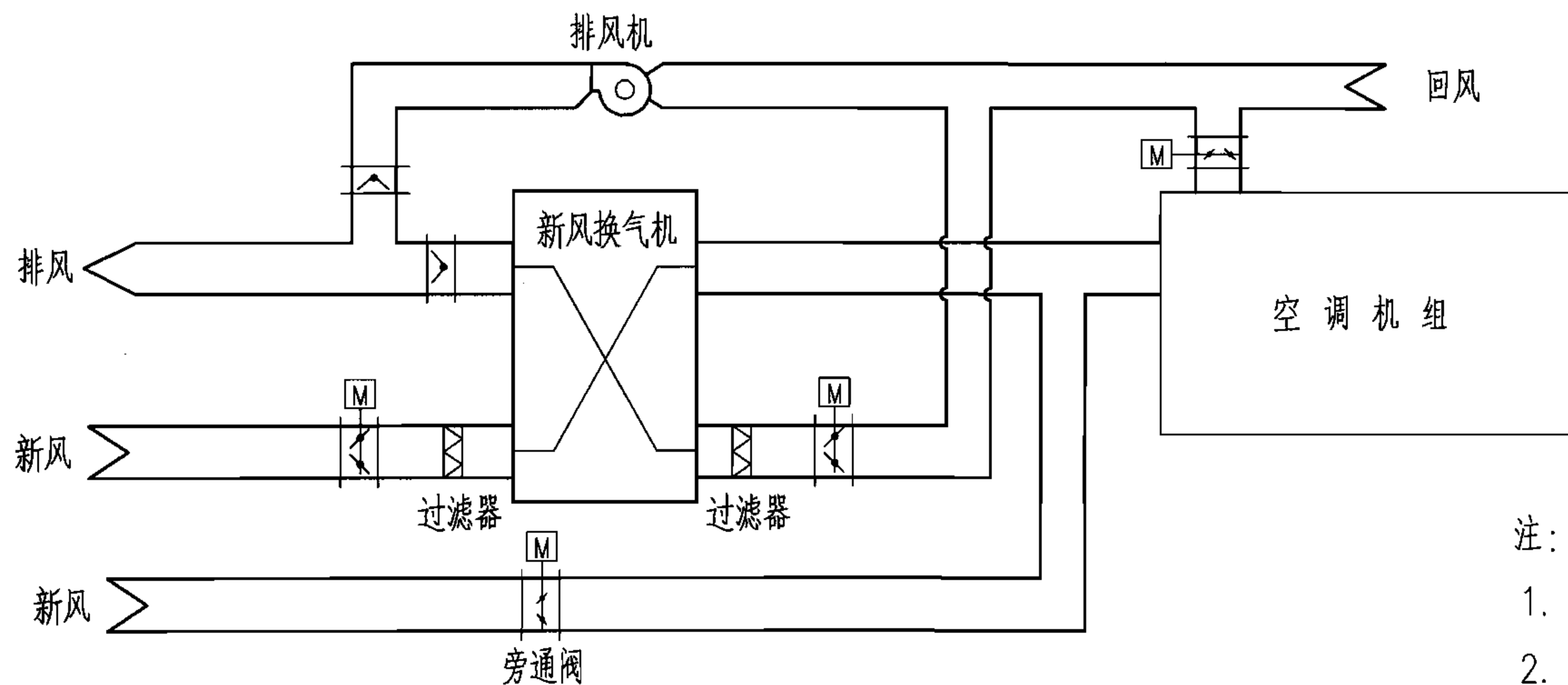
系统流程图
