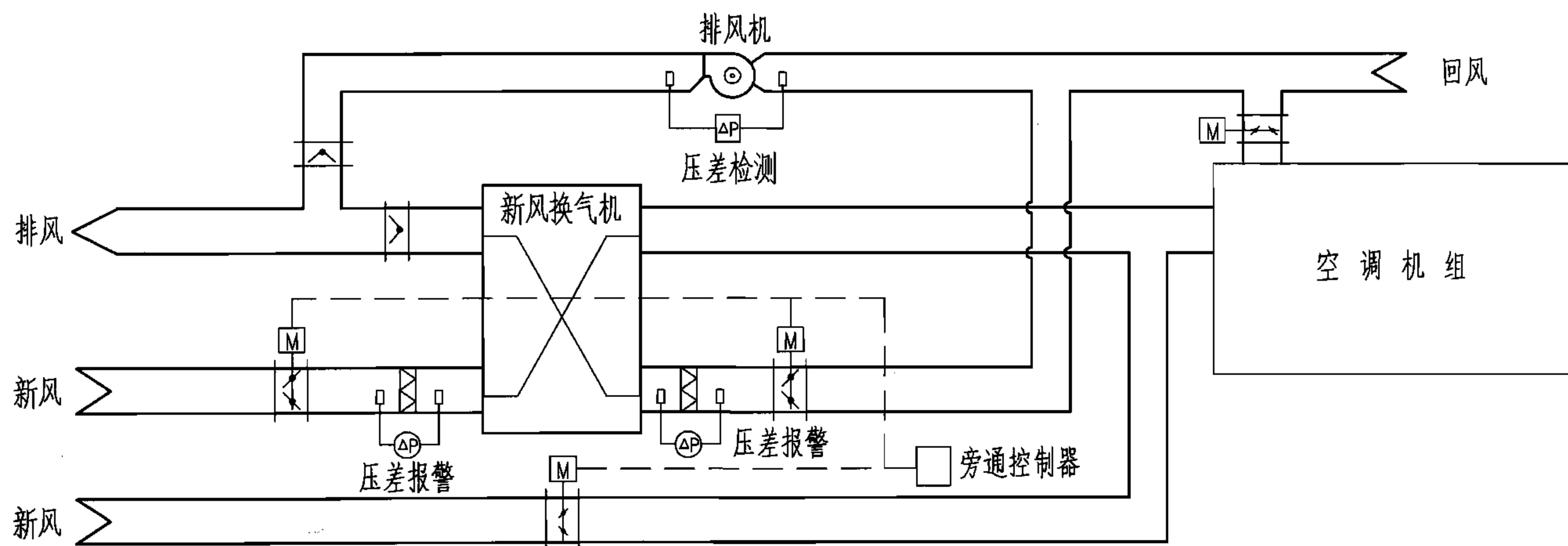
控制原理图
