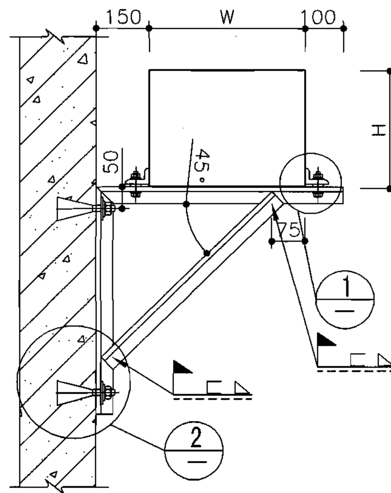
钢筋混凝土墙上安装
