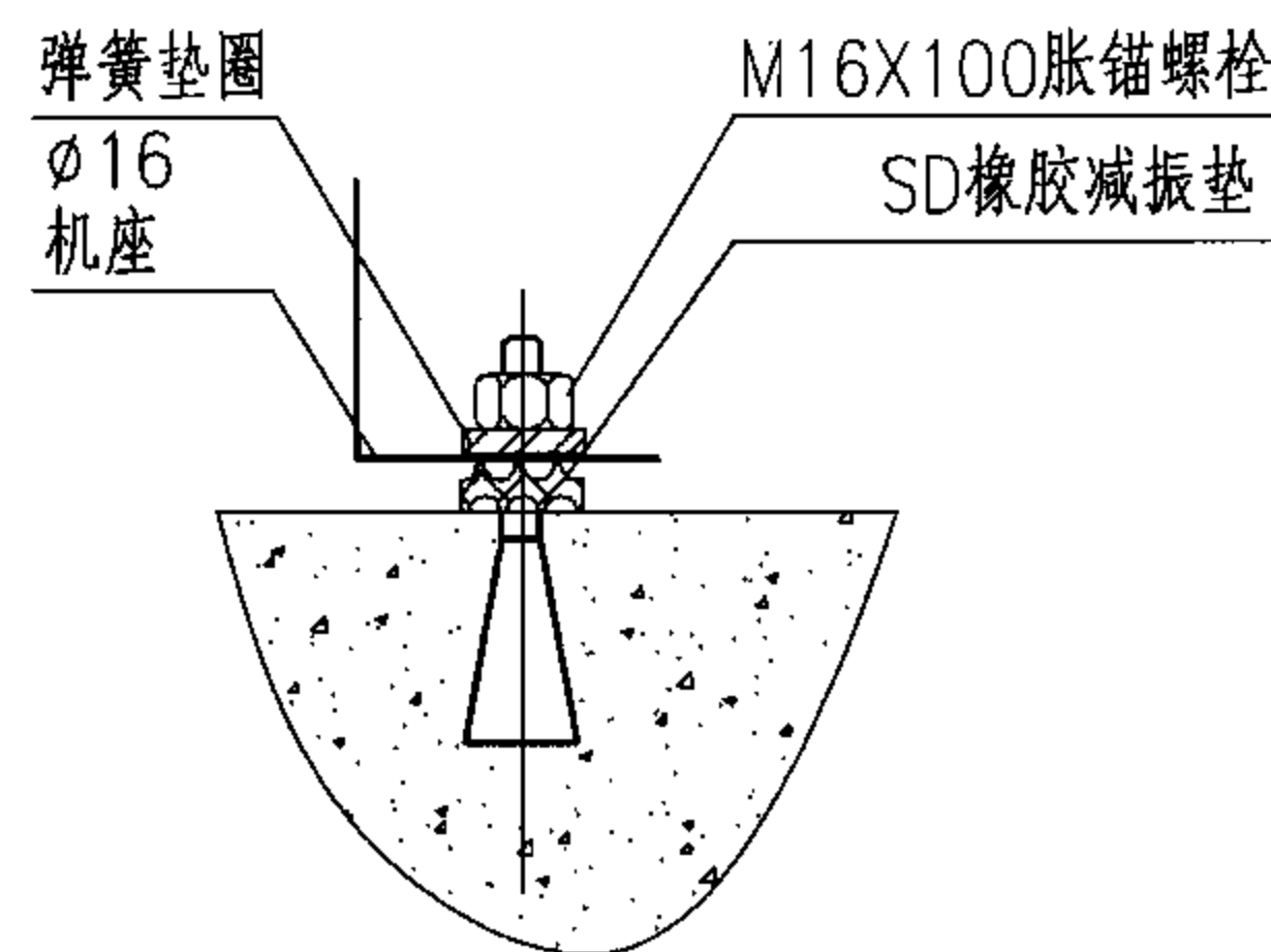
SD橡胶减振垫安装
