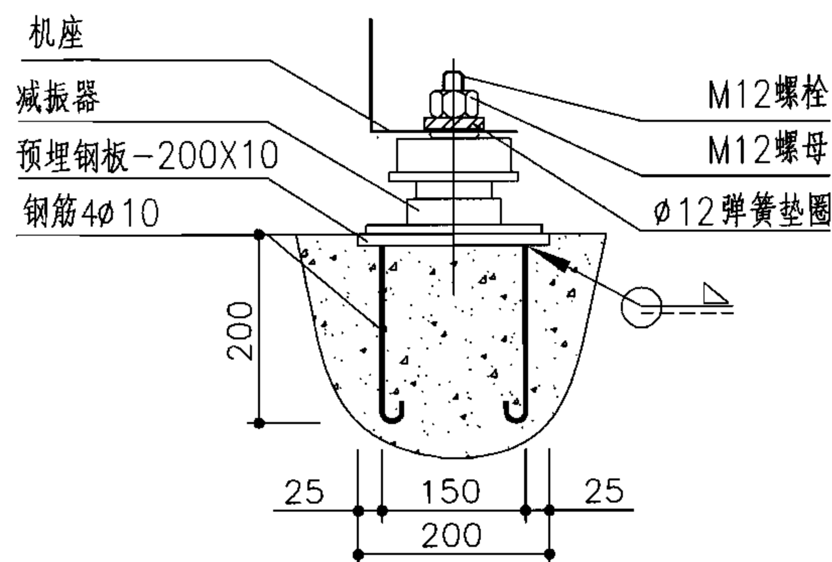
弹簧减振器安装
